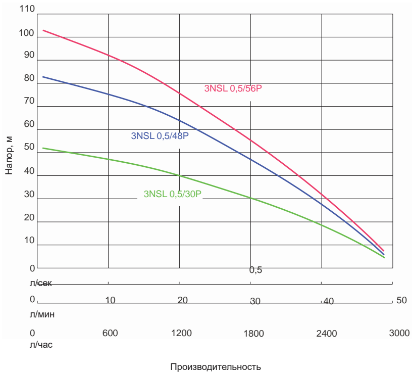
График производительности
