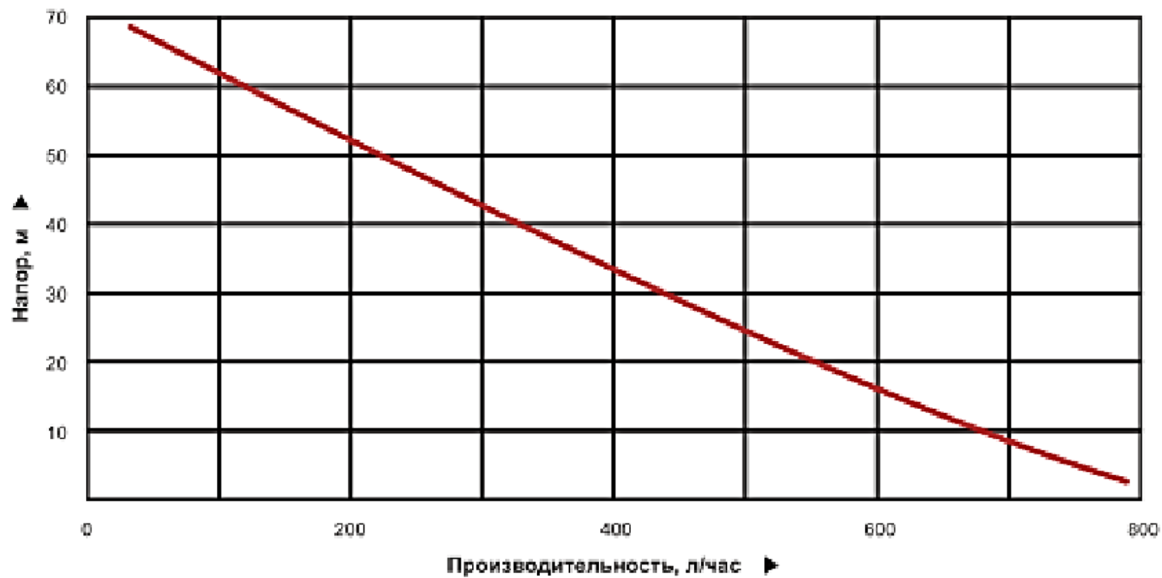
График производительности вибрационных насосов серии БВ
