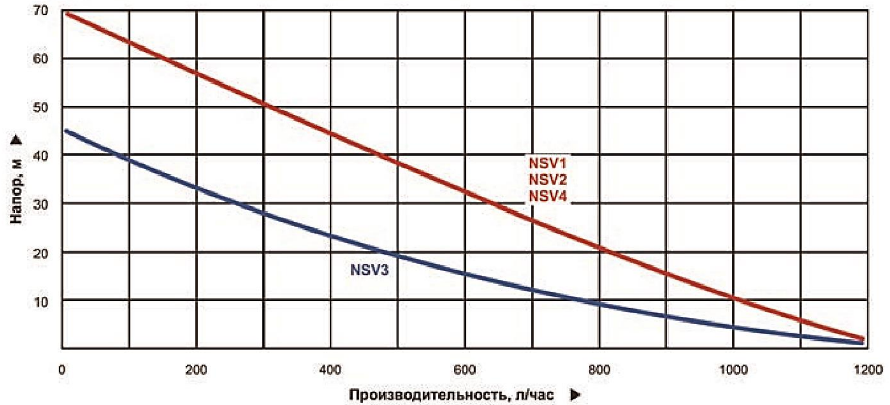
График производительности вибрационных насосов WWQ серии NSV
